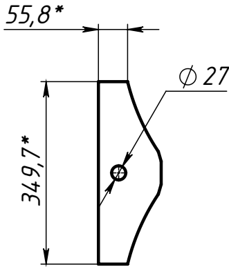
Поз.3 (Ушко) развертка
